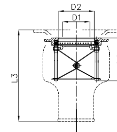
Prise femelle / Mutterstück
