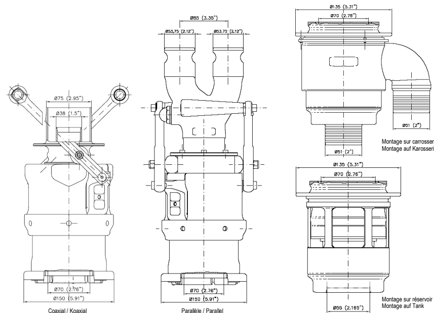
Dessin/Skizze 252-5 (Version B) (Accoupleur mâle / Kupplung männlich)
