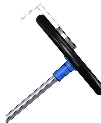
DESSIN TECHNIQUE N°1.2
