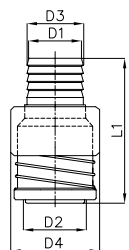
Prise mâle / Steckstück
