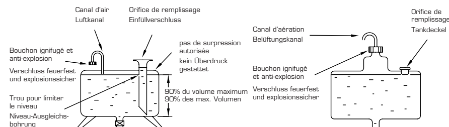
Dessin/Skizze 252-3
