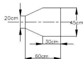
Dessin/Skizze 259-2
