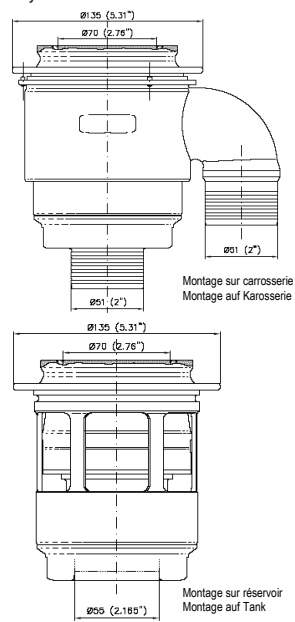
Dessin/Skizze 252-5 (Version B) (Accoupleur femelle / Buchsenkupplung)
