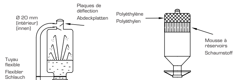
Dessin/Skizze 252-2
