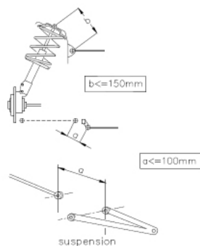
Dessin/Skizze 255-4
