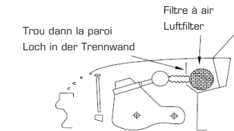
Dessin/Skizze 255-6
