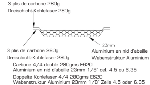
Dessin/Skizze 255-14
