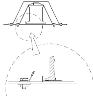
Dessin/Skizze 255-11
