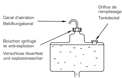
Dessin/Skizze 252-4
