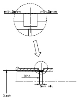
Dessin/Skizze 254-4
