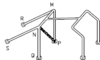
Dessin/Skizze 259-3
