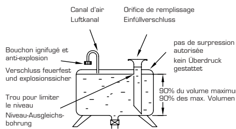
Dessin/Skizze 252-3
