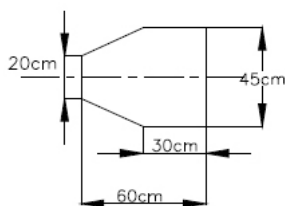
Dessin/Skizze 259-2
