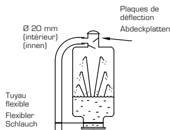
Dessin/Skizze 252-1
