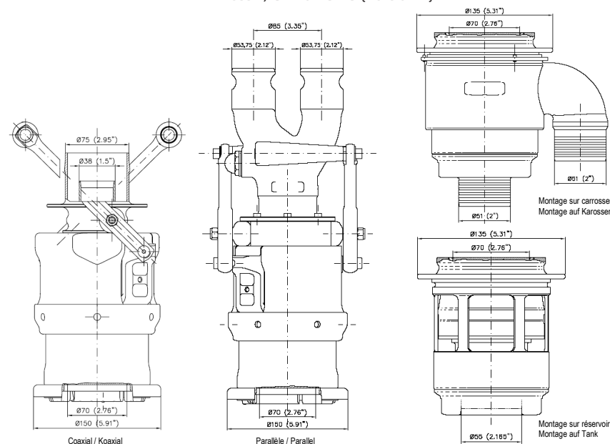
Dessin/Skizze 252-5 (Version B) (Accoupler mâle / Kupplung männlich)
