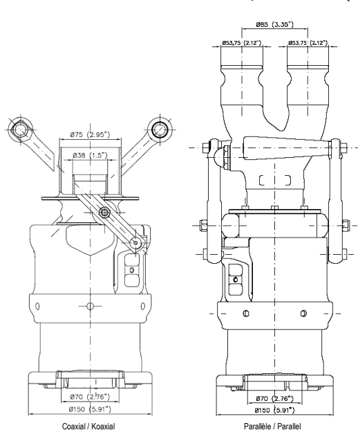
Dessin/Skizze 252-5 (Version B) (Accoupleur mâle / Steckerkupplung)
