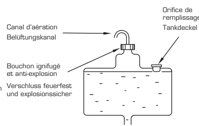
Dessin/Skizze 252-4
