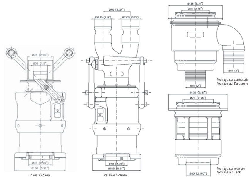
Dessin/Skizze 252-5 (Version B) (Accoupler mâle / Steckerkupplung)
