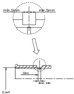
Dessin/Skizze 254-4
