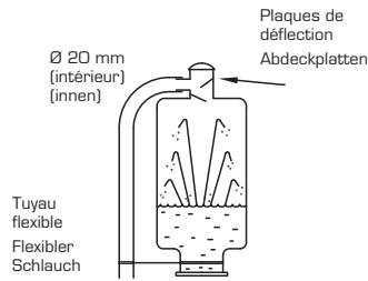
Dessin/Skizze 252-1
