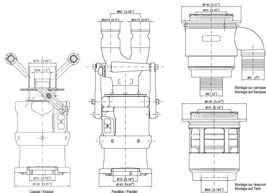
Dessin/Skizze 252-5 (Version B) (Accoupleur mâle / Steckerkupplung)
